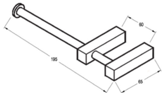
Dimensions
