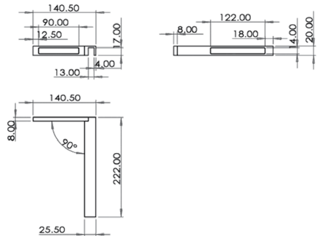
Dimensions
