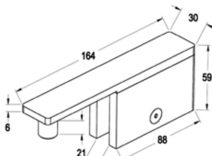
Dimensions
