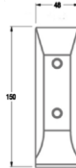
Dimensions
