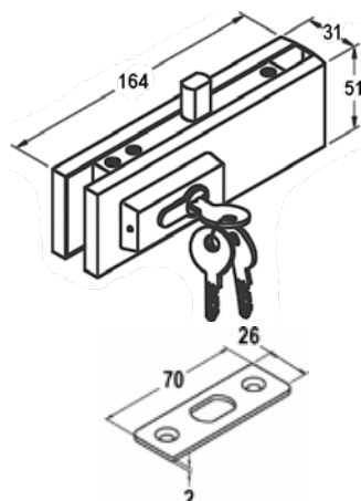
Dimensions
