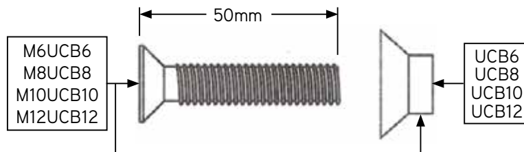
Dimensions
