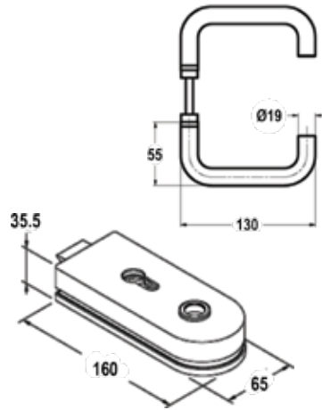
Dimensions
