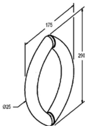
Dimensions
