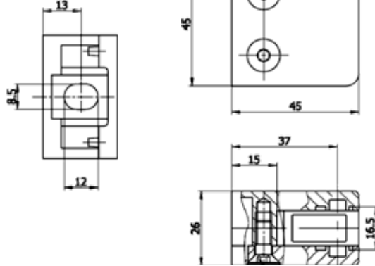
Dimensions
