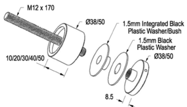
Dimensions
