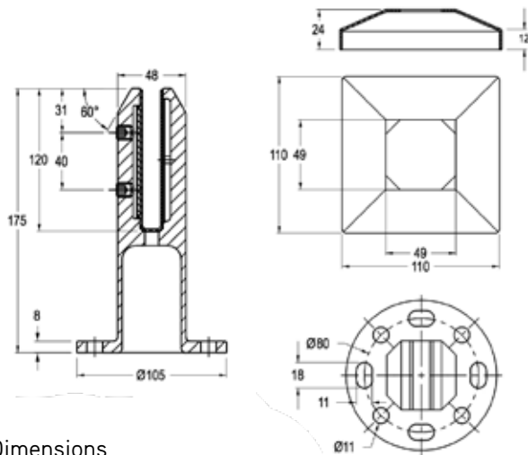
Dimensions
