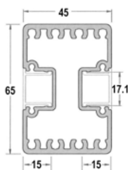
Dimensions
