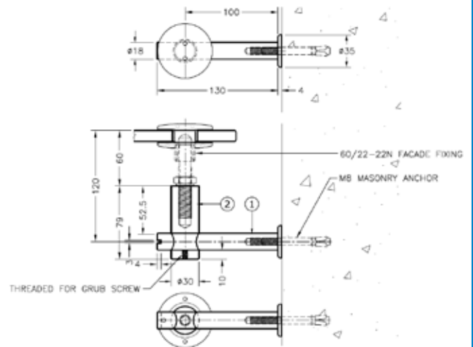
Dimensions
