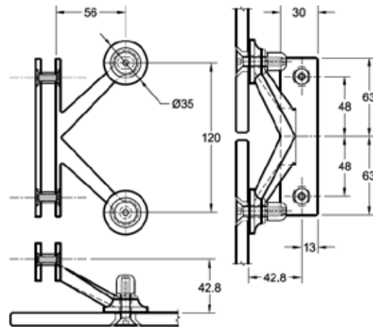
Dimensions
