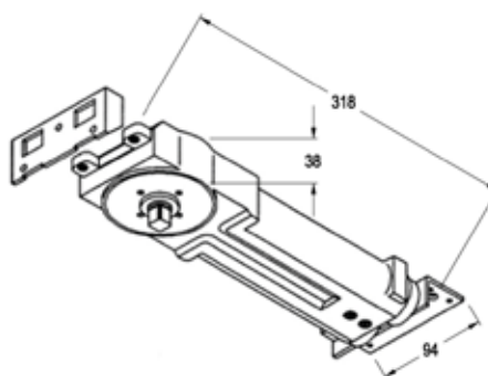
Dimensions
