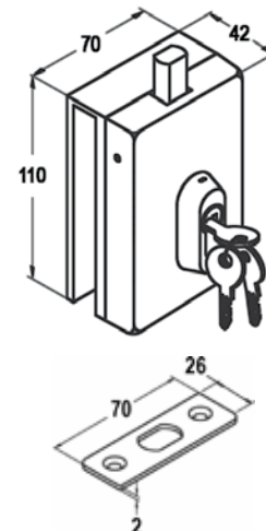
Dimensions
