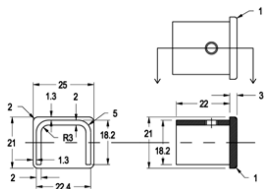
Dimensions
