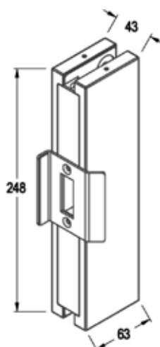
Dimensions
