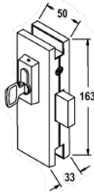
Dimensions
