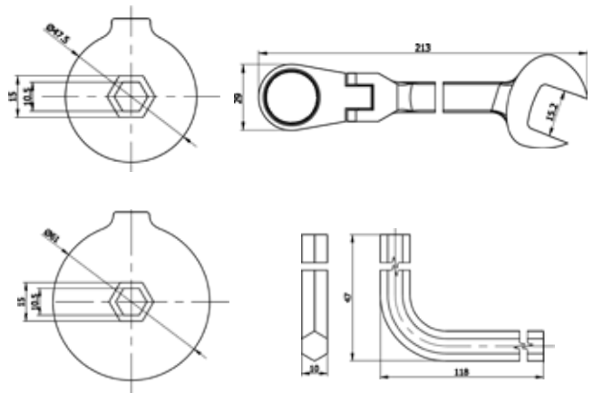
Dimensions
