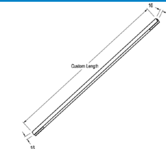
Dimensions
