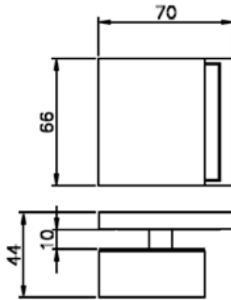
Dimensions
