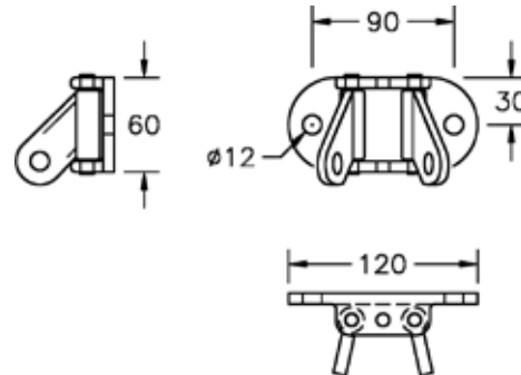
Dimensions
