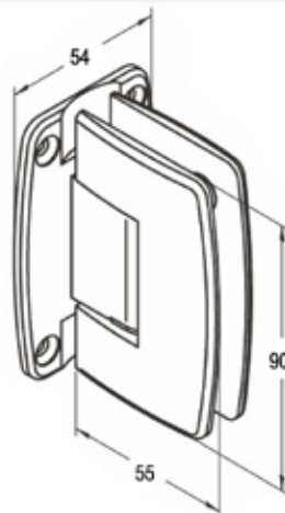
Dimensions
