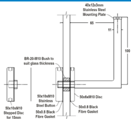
Dimensions
