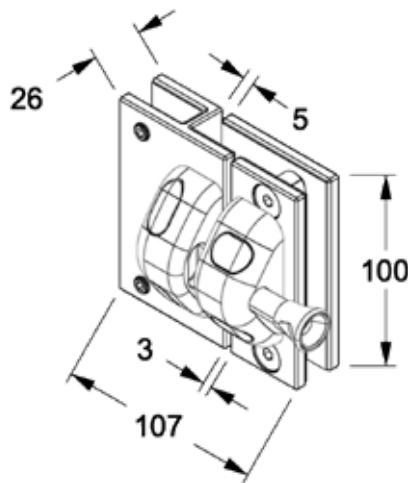
Dimensions
