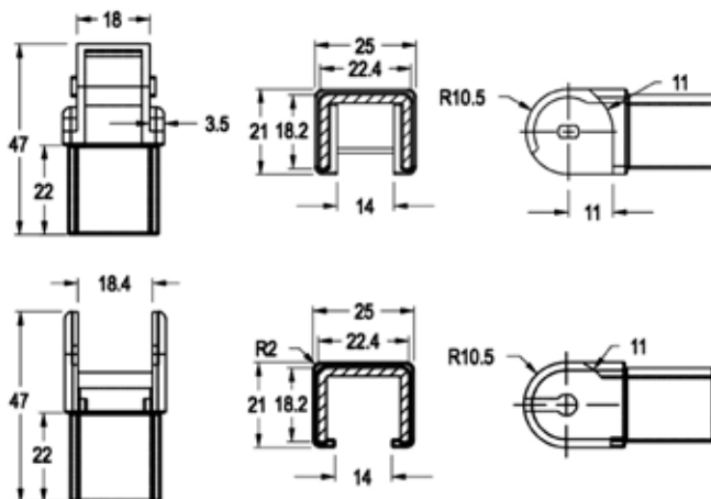
Dimensions
