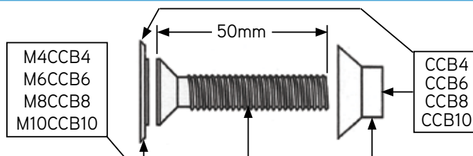
Dimensions
