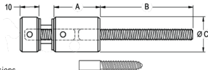
Dimensions
