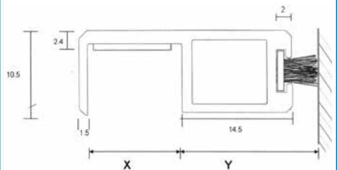
Dimensions
