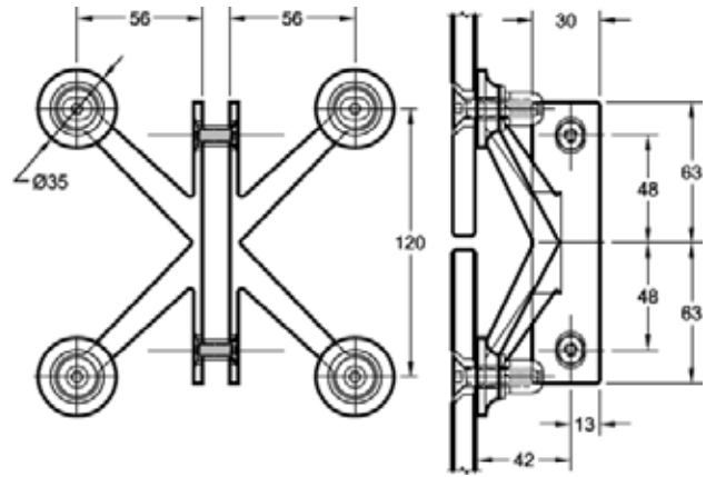
Dimensions
