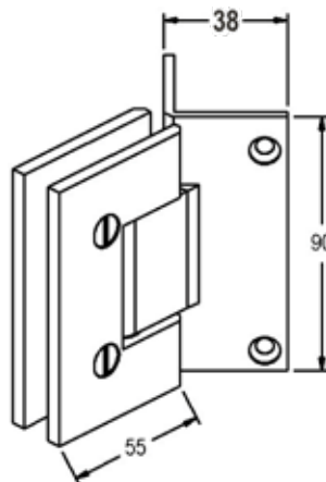
Dimensions
