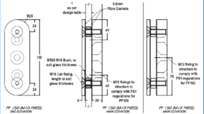
Dimensions
