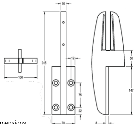
Dimensions
