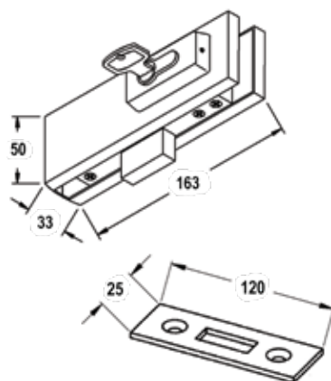
Dimensions
