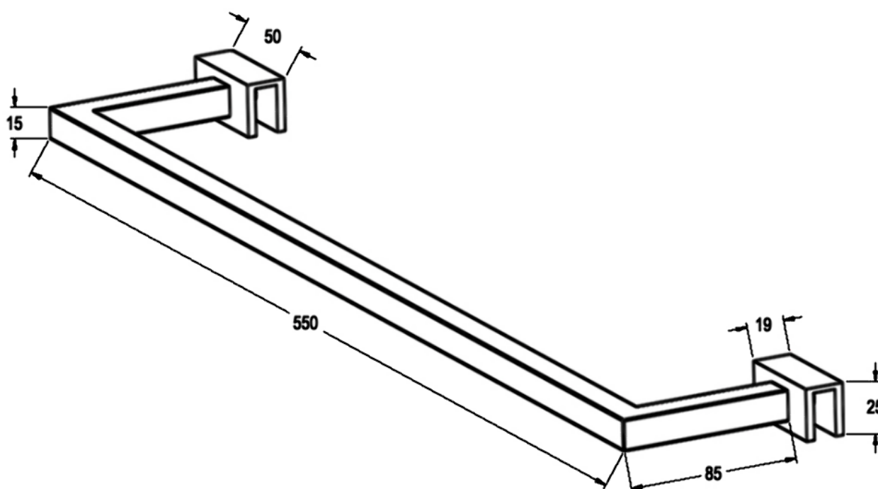
Dimensions
