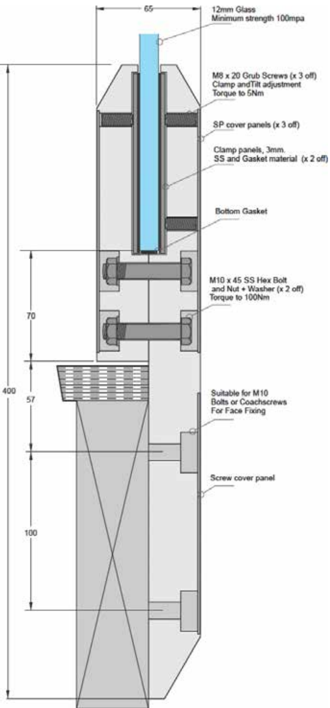
Dimensions
