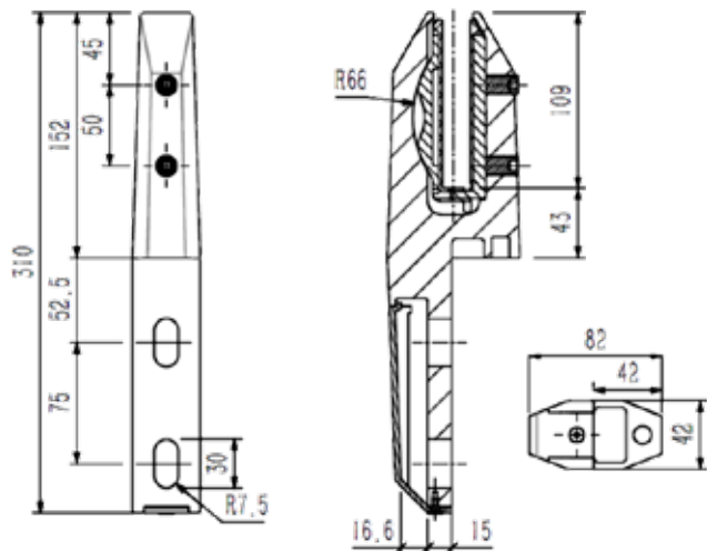
Dimensions
