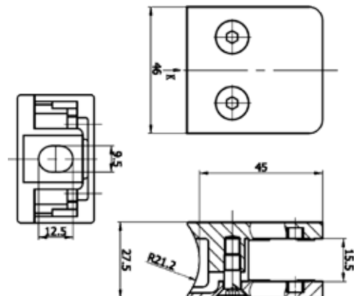
Dimensions
