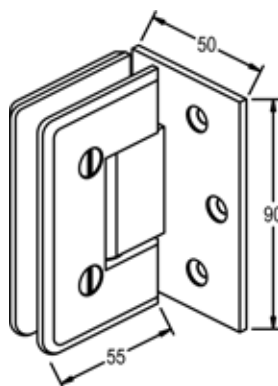
Dimensions
