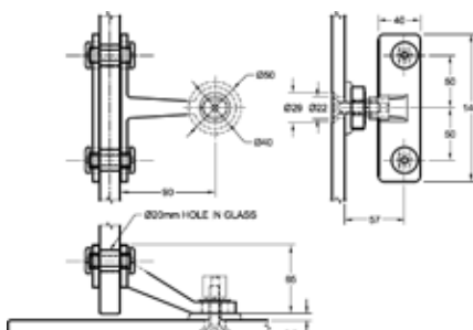
Dimensions
