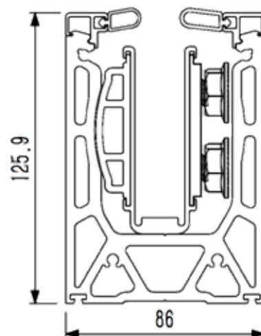
Dimensions
