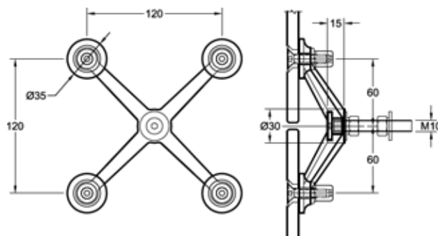
Dimensions
