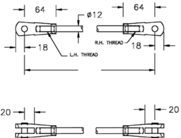
Dimensions
