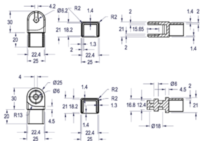
Dimensions
