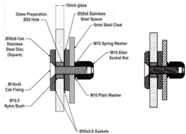
Dimensions
