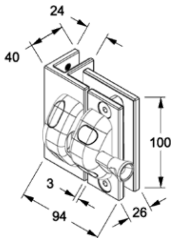
Dimensions
