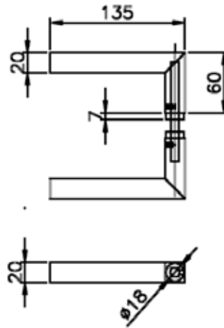
Dimensions
