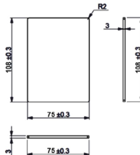
Dimensions
