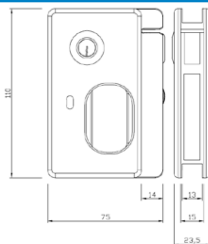
Dimensions
