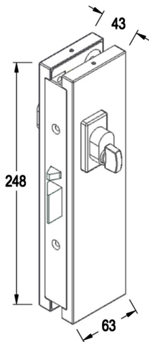
Dimensions
