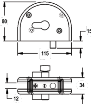
Dimensions
